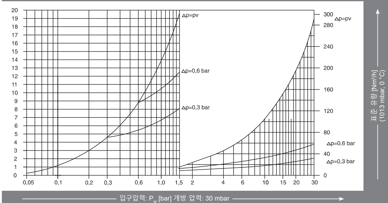
유량표 (대기 기준, 20 °C)
